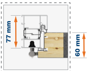
ALUTHERM 60* door frame
