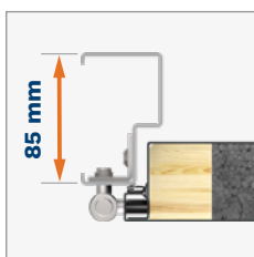
FB steel door frame
