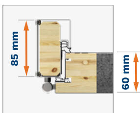
DUOTHERM 60 door frame
